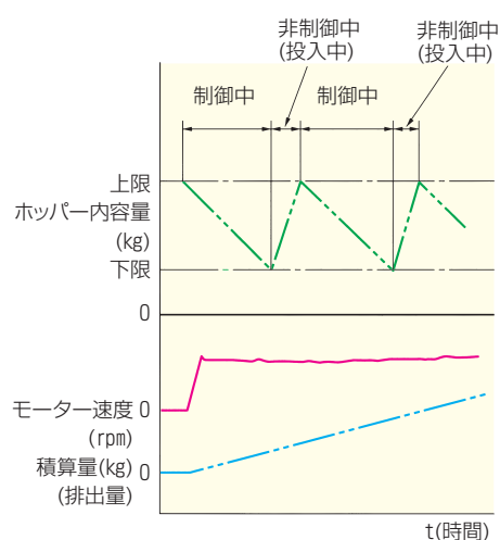
動作図
