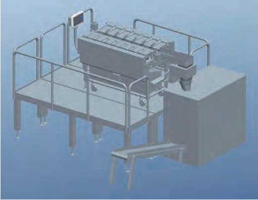
包装機との連動
